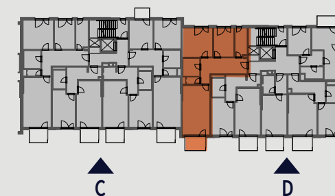
Půdorys podlaží | Floor Plan
